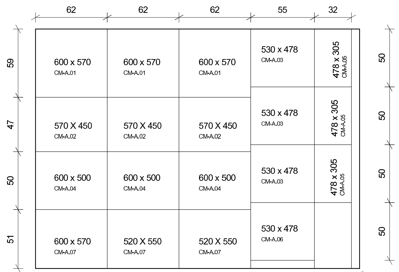
DEBIT POUR 3 CAISSONS MOBILE A
