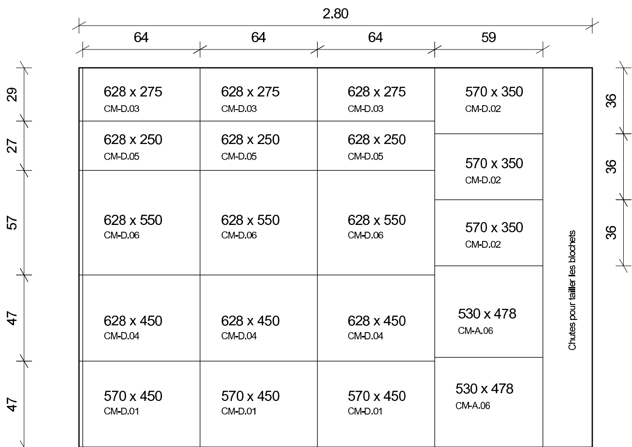
DEBIT POUR 3 CAISSONS MOBILE D
