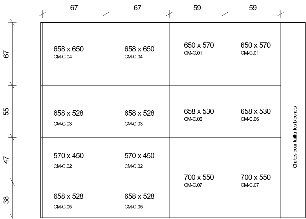
DEBIT POUR 2 CAISSONS MOBILE C
